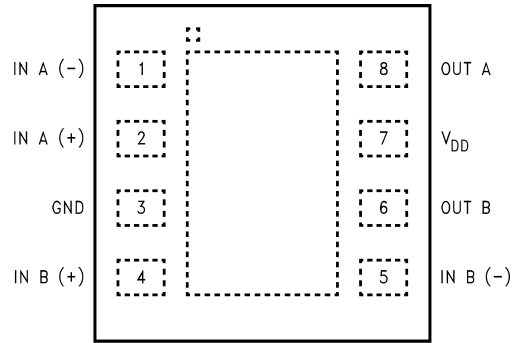
LLP Package
